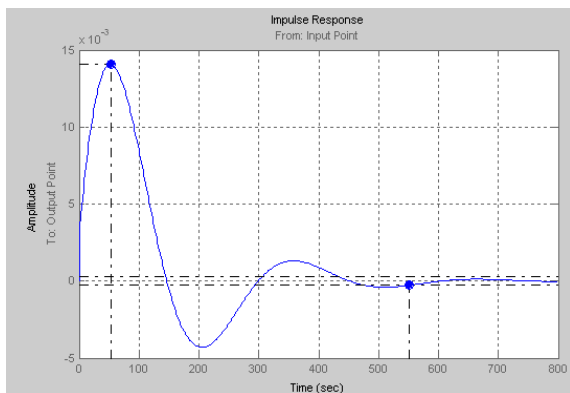
Импульсная функция
