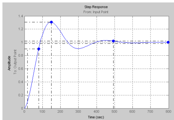
Переходная функция
