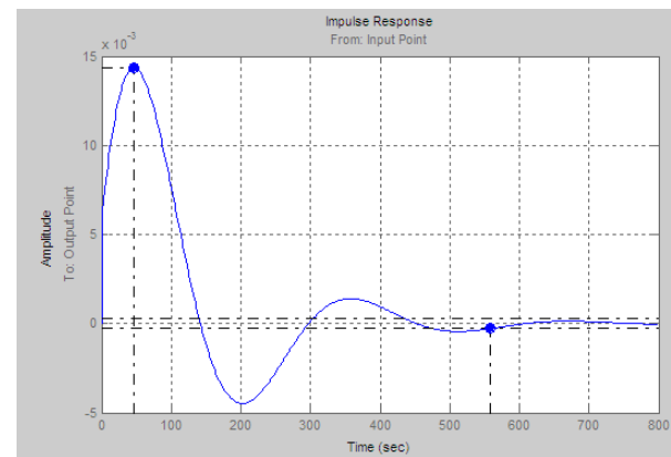
Импульсная функция
